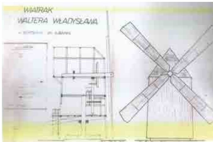
Rysunek przedstawiający elementy pierwotnej konstrukcji wiatraka
